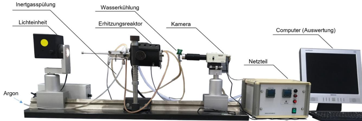
Messapparatur von Hesse Instruments (EM201 von E. Leitz Wetzlar)
