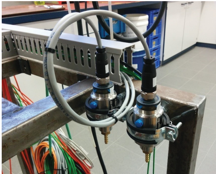
Abbildung 8: Pellet-Pot – Drucksensoren
