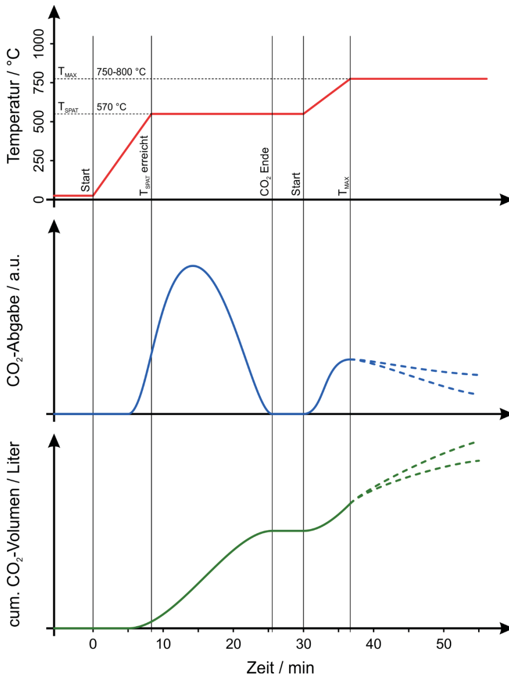
Abbildung 25: Erzcharakterisierung – Geplanter Versuchsablauf
