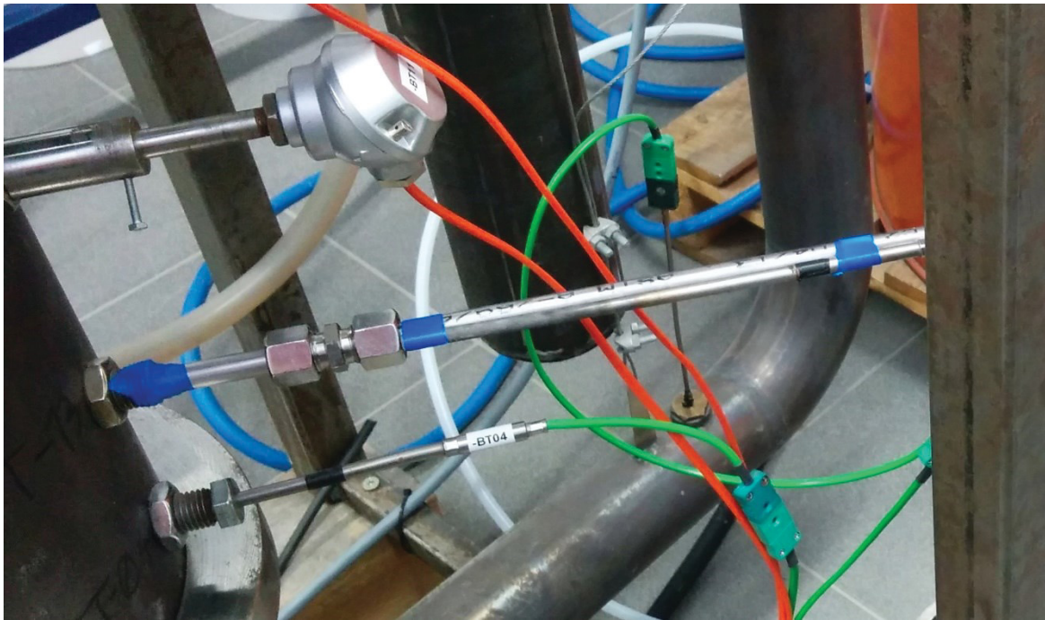
Abbildung 31: Gasmessstrecke – Austritt der Messleitung aus dem Pot
