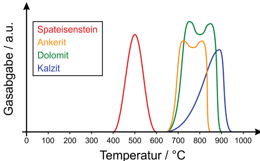
Abbildung 24: Erzcharakterisierung – Gasabgabebereiche der relevanten Karbonate
