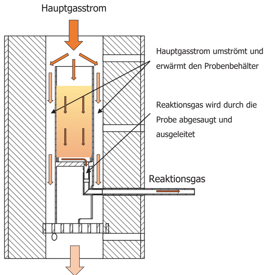
Abbildung 28: Probenbehälter – Funktionsprinzip
