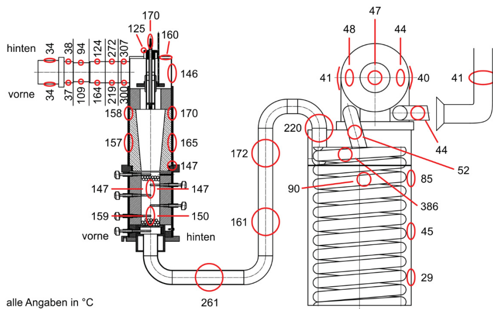
Abbildung 23: Inbetriebnahme – Maximale Oberflächentemperaturen am Pellet-Pot
