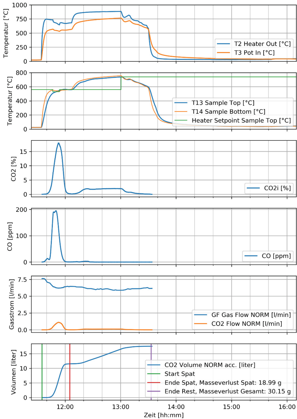
Abbildung 41: PPV-007-IB „Kleine Probenmenge“ – Versuchsablauf
