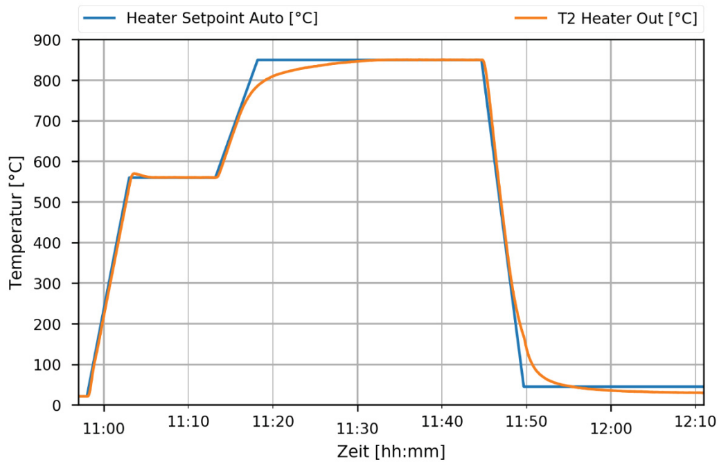
Abbildung 20: Inbetriebnahme – Automatikmodus – Test 2 – Temperaturvergleich
