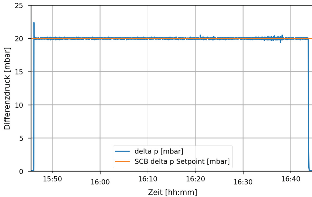
Abbildung 18: Inbetriebnahme – Automatikmodus – Test 1 – Differenzdruckverlauf
