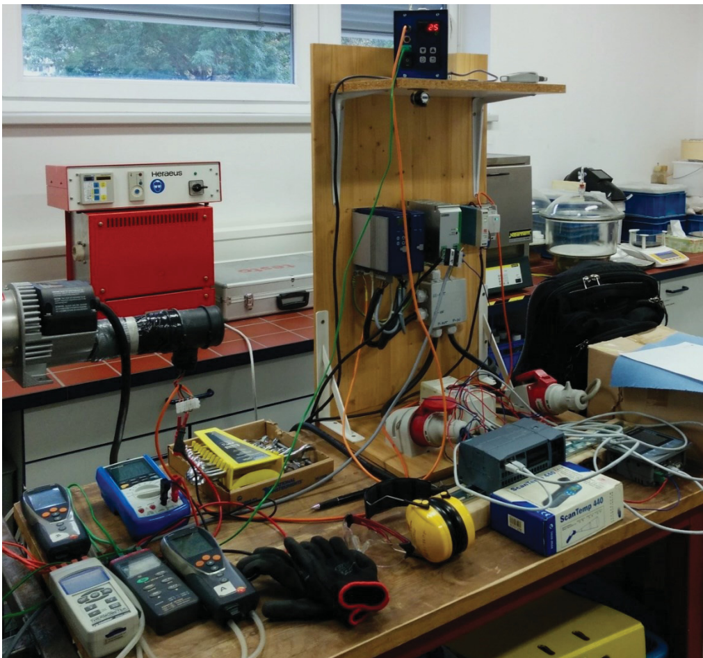
Abbildung 5: Pellet-Pot – Ausgangssituation – Elektrik und Messtechnik
