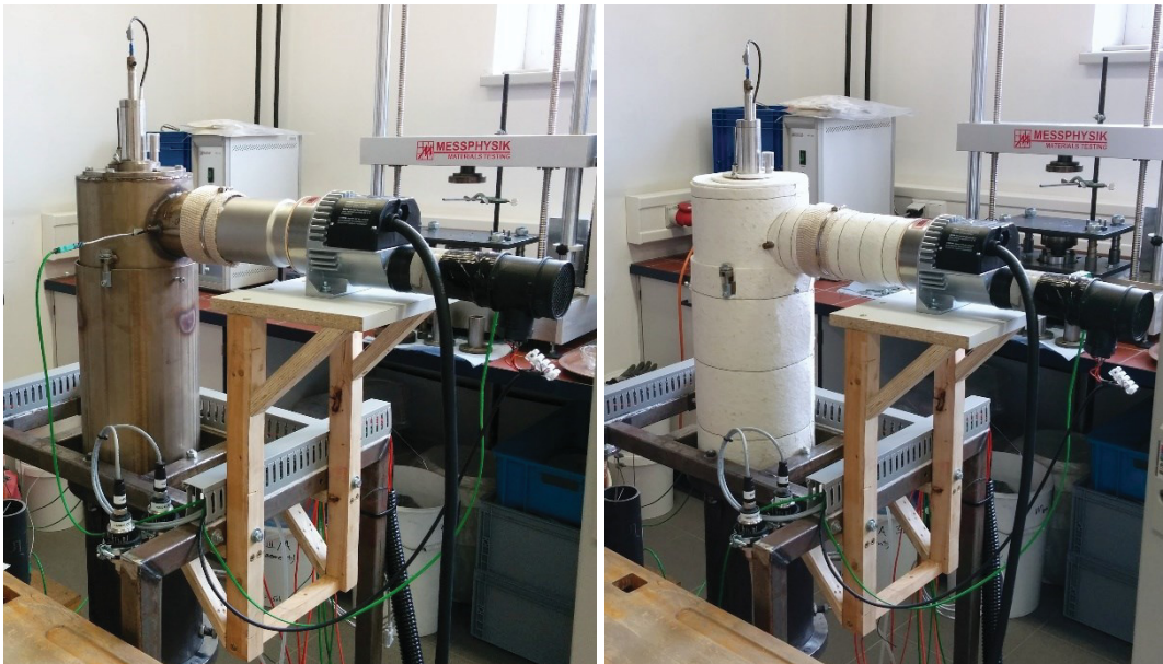
Abbildung 10: Pellet-Pot – ungedämmt/gedämmt
