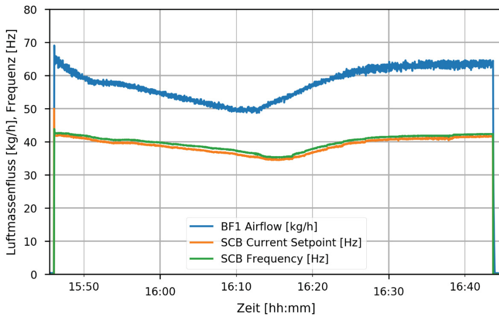
Abbildung 19: Inbetriebnahme – Automatikmodus – Test 1 – Differenzdruckregelung
