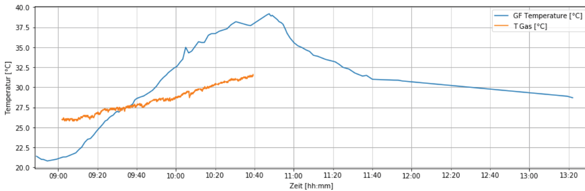
Abbildung 32: Gasmessung – Vergleich Gastemperaturen – Temperatur Messgerät (orange), Temperatur Messgasstrom (blau)
