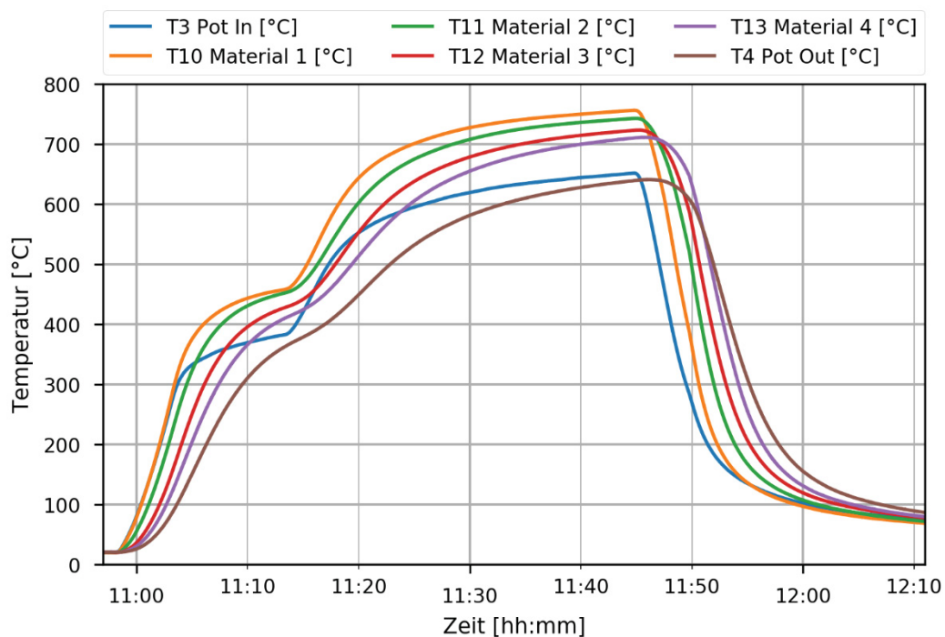
Abbildung 21: Inbetriebnahme – Automatikmodus – Test 2 – Temperaturen im Pot
