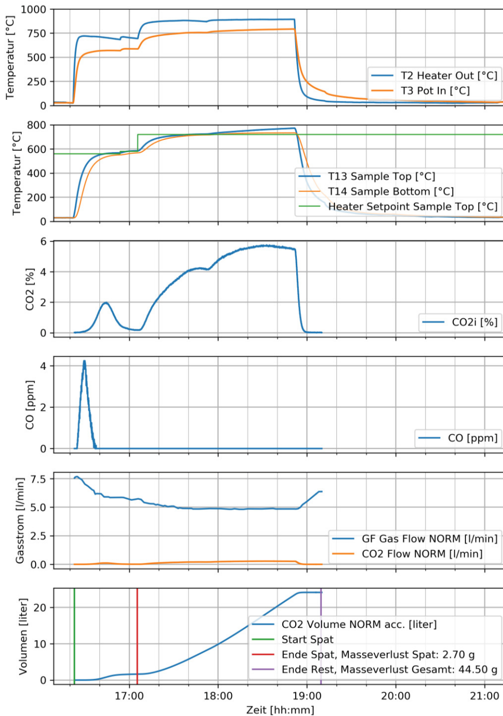
Abbildung 40: PPV-006-IB „Ankeritstandard“ – Versuchsablauf
