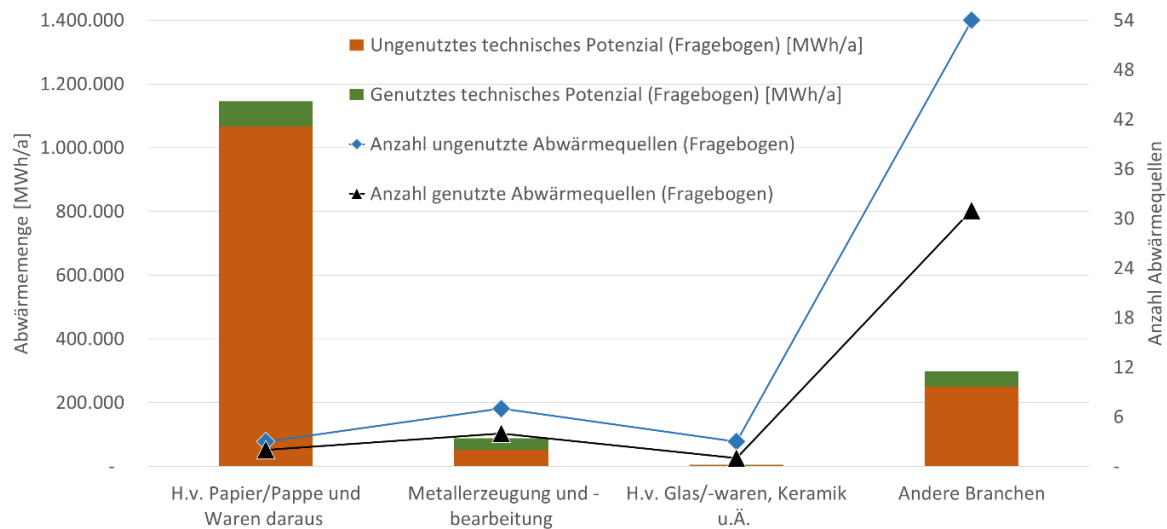
Abbildung 4: Ungenutztes und genutzte technische Potenziale aus der Fragebogen Erhebung und Anzahl der Abwärmequellen.
