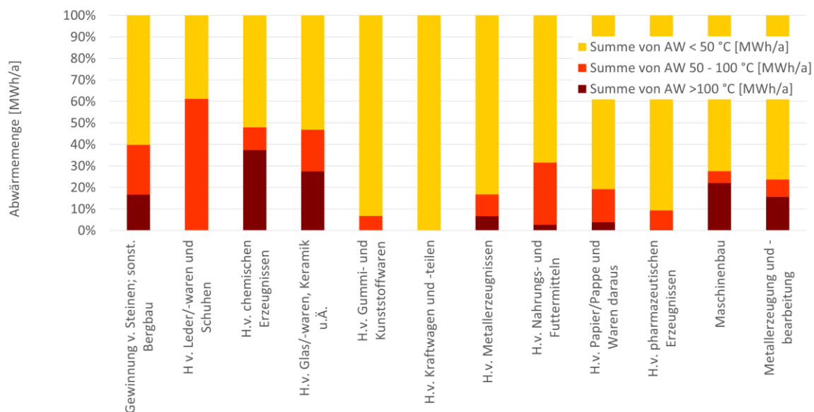
Abbildung 7: Prozentuelle Aufteilung nach Temperaturkategorien des technischen Abwärmepotenzials (ungenutzt+genutzt) der Abwärmquellen für ausgewählte Branchen (mind. 10.000 MWh/a technisches Abwärmepotenzial).
