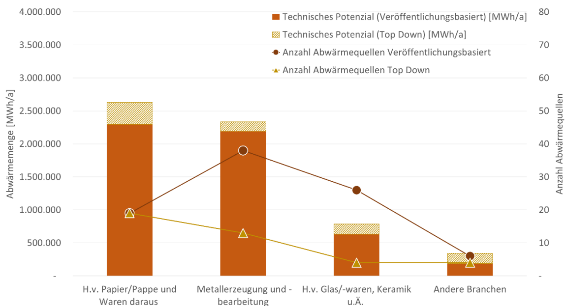
Abbildung 5: Technische Potenziale aus Top Down und veröffentlichungsbasierter Erhebung. Angaben in MWh/a. Anzahl der Abwärmequellen pro Erhebungsmethode. Gesamtpotenziale (ungenutzt+genutzt).
