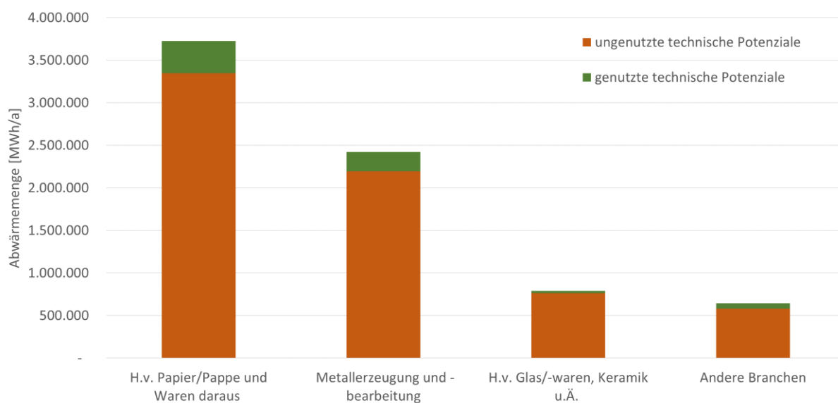
Abbildung 2: Branchenübersicht der ungenutzten und genutzten technischen Potenziale in MWh/a. Andere Branchen umfasst alle nicht separat ausgewiesenen Branchen (Details in Tabelle 2).
