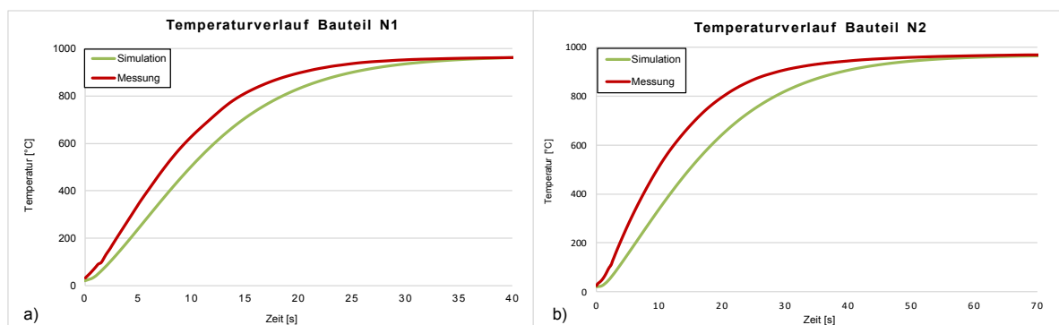
Abbildung 4.10: Vergleich der Temperaturverläufe von Simulation und Messung
