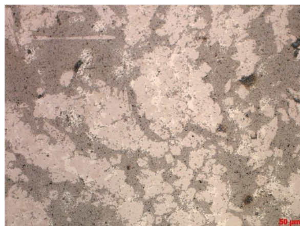
675 °C, 15 % Co, KG: M, 2 h – 100-fach
