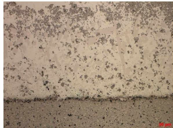
675 °C, 12 % Co, KG: G, 0,5 h – 100-fach
