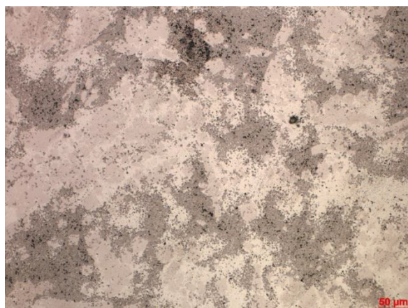
675 °C, 12 % Co, KG: M, 2 h – 100-fach
