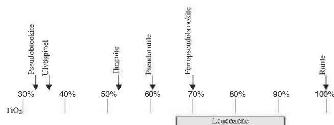
Abb. 11: Theoretischer \text{TiO}_2 -Gehalt in FeTi-Oxidphasen (Gew. %), mit FeO und \text{Fe}_2\text{O}_3 als zweite Endglieder in diesem binären System (Reyneke & Wallmach, 2007).
