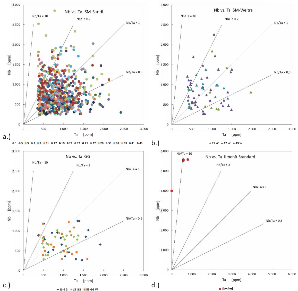
Abb. 39 a-d: Nb gegen Ta Diagramme mit Nb/Ta-Verhältnissen (Linien). Dargestellt sind nur Analysen für die sowohl die Nb als auch die Ta-Werte über der Nachweisgrenze liegen (siehe Tab. 5).
