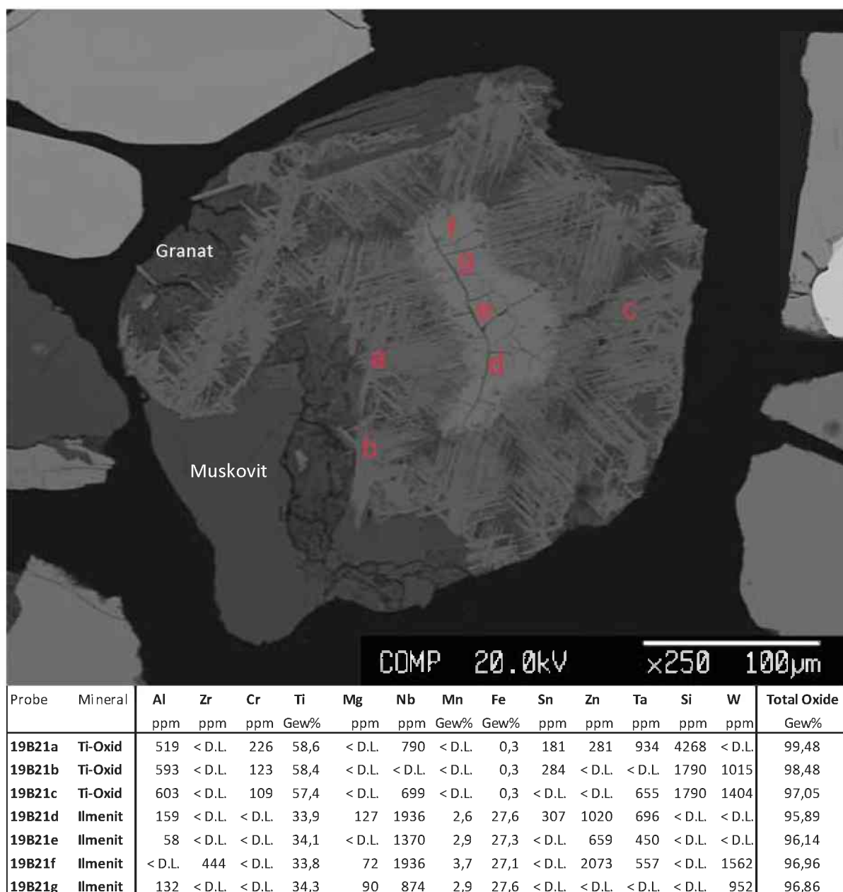
Abb. 29: Rückstreuerelektronen-Bild eines polyphasen Kornes der Probe 19B21 mit Messpunkten und dazugehöriger Ergebnistabelle. Titanoxid (Rutil?) mit sagenitischer Struktur (a-c), Ilmenit im Kornkern (d-g) mit Schrumpfungsrissen sowie Muskovit und Granat. (< D.L. = unter der Nachweisgrenze).
