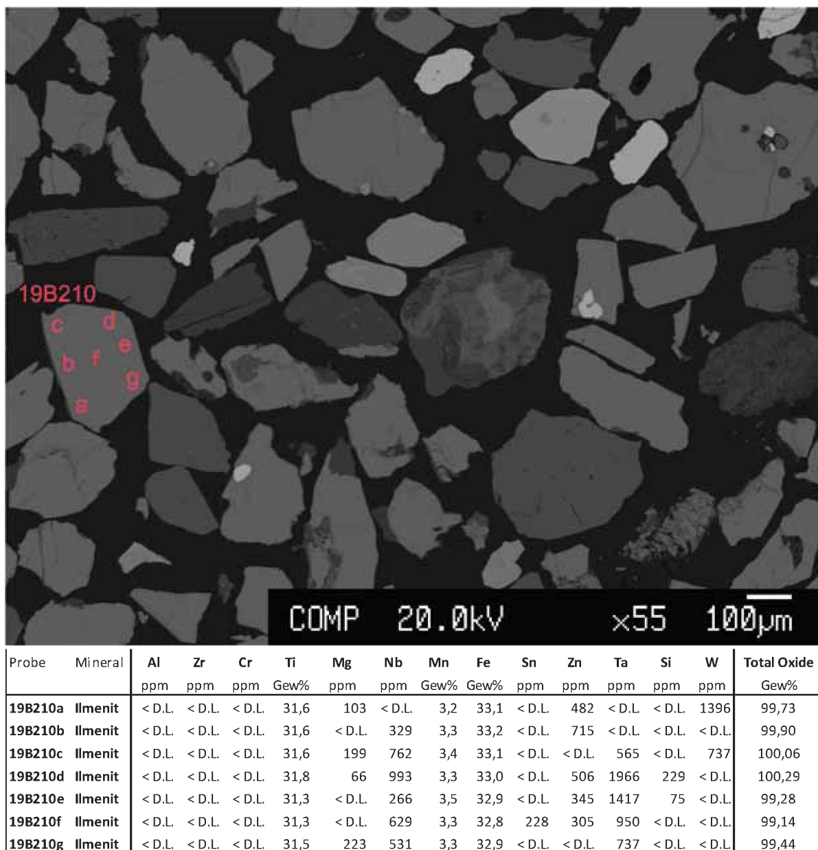
Abb. 26: Rückstreuelektronen-Bild eines monomineralischen Ilmenitkorns mit der Messbezeichnung 19B210 samt Messpunkten und dazugehöriger Ergebnisstabelle. (< D.L. = unter der Nachweisgrenze)
