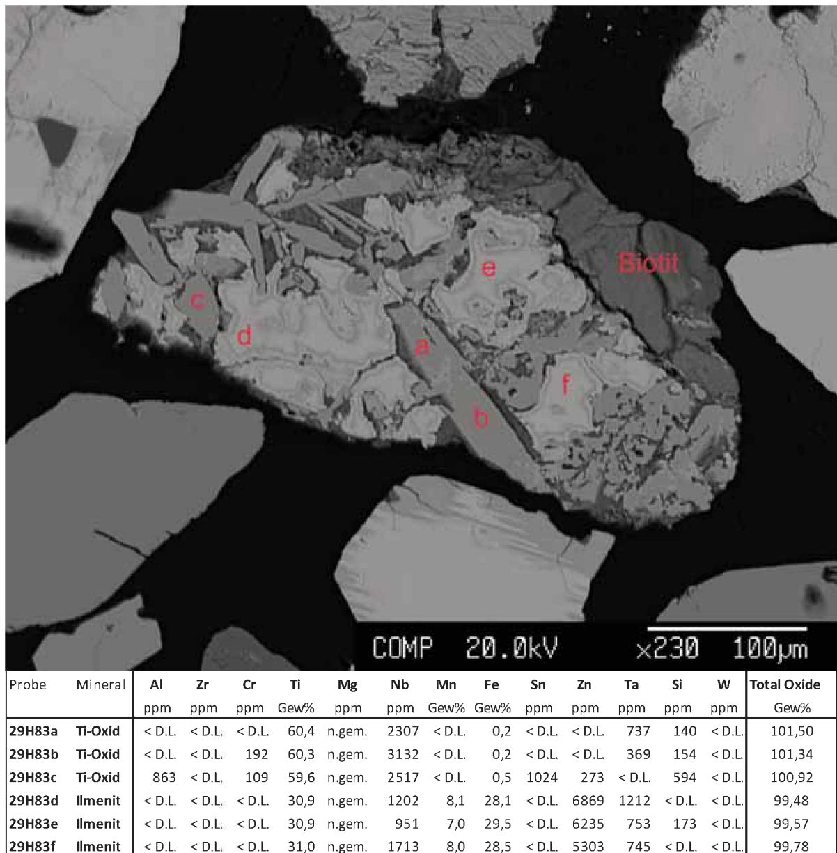
Abb. 28: Rückstreuelektronen-Bild eines polyphasen Kornes bestehend aus Titanoxid, Ilmenit und Biotit der Probe 29H83 mit Messpunkten und dazugehöriger Ergebnistabelle (< D.L. = unter der Nachweisgrenze; n.gem. = nicht gemessen).
