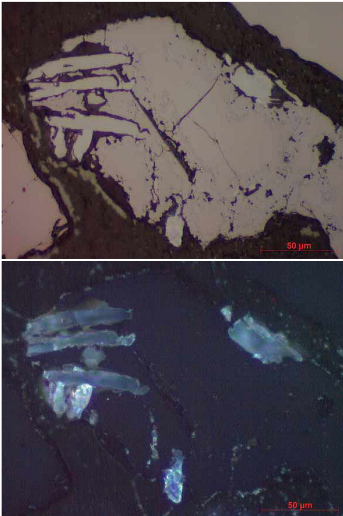
Abb. 14: Ilmenit verwachsen mit hypidomorphem Anatas (unteres Bild +N: bläulich) und Fe-Abfuhr in den grünlischen Randbereichen; 50fache Vergrößerung, Nicols parallel (oben) und gekreuzt (unten), Probe 07A13 (07A13-Ilm+Rut_50IIN).
