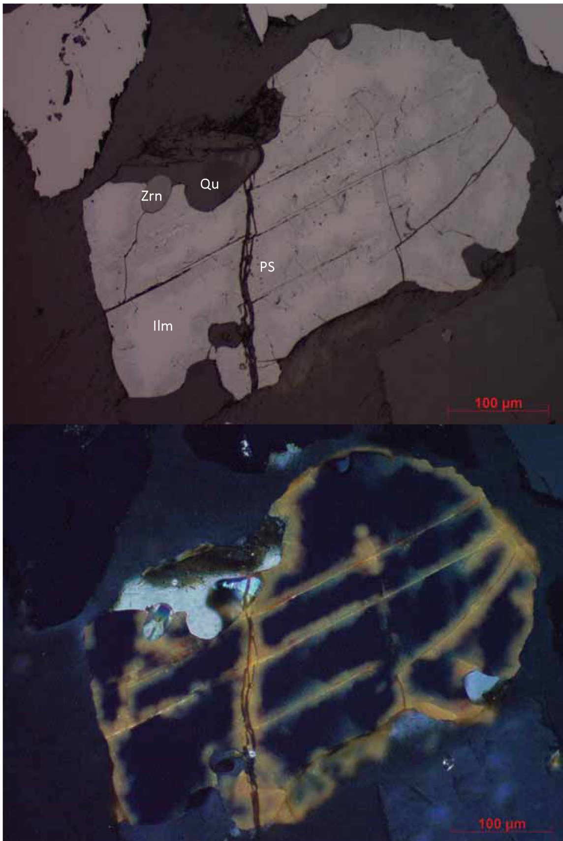
Abb. 15: Ilmenitkorn mit drei Titan-Phasen: Nicht alterierter Ilmenit (//N, Bild oben, braungrau, Ilm) mit Umwandlung in Pseudorutil entlang von Rissen (//N, Bild oben, grau-blau, PS) und in Leucoxen in den Rissen (+N, Bild unten, gelblich). Einschluss von Zirkon (Zrn) und Verwachsung mit Quarz (Qu). (20fache Vergrößerung, oben //N, unten +N, Probe 03)
