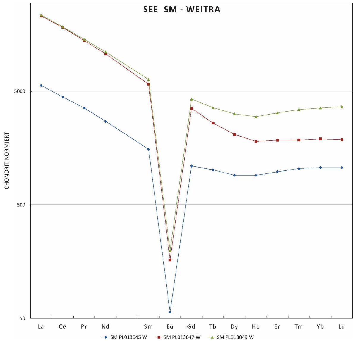
Abb. 53: SEE-Verteilung der SM-Proben aus dem Raum Weitra (LREE – HREE), in logarithmischer Darstellung, Chondrit-normiert (nach Wasson & Kallemeyn, 1988).
