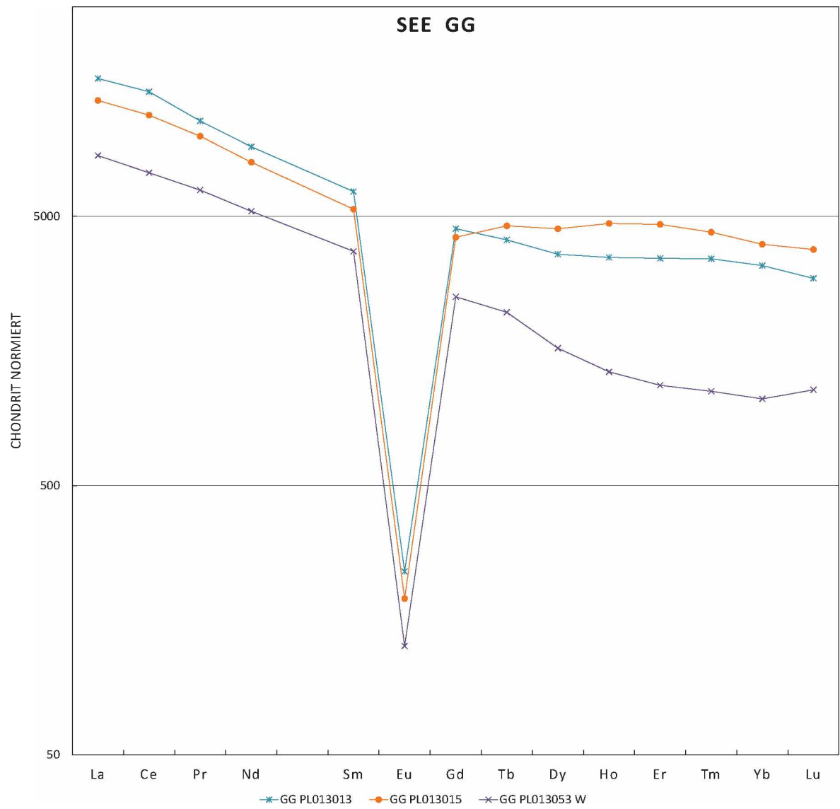
Abb. 54: SEE-Verteilung der GG-Proben in logarithmischer Darstellung, Chondrit-normiert.
