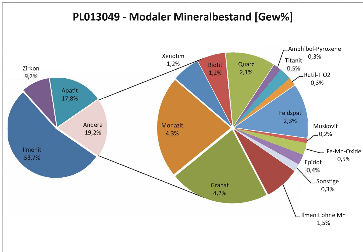
u.) SM Probe, Weitra
