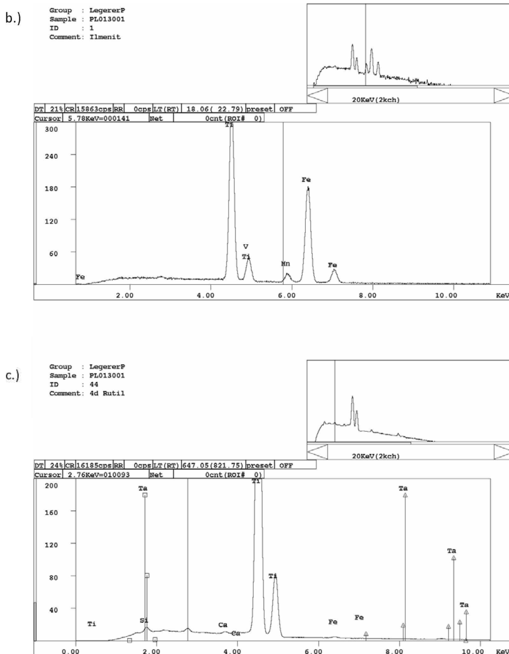
Abb. 24 a-c: EDS-Spektren von Titanit, Ilmenit und Titanoxid ( \text{TiO}_2 ), Marker-Linien zeigen Position elementspezifischer L bzw. M-Linien von Nb bzw. Ta.
