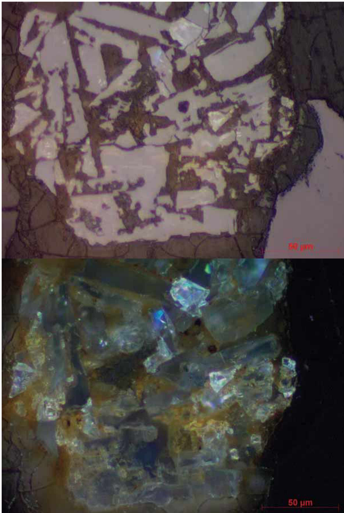
Abb. 19: Vorwiegend in Anatas (+N: bläulich) und Leucosin (+N: gelblich) umgewandelter Ilmenit. Auflicht, 50fache Vergrößerung, Nicols parallel (oben) und gekreuzt (unten), Probe05C31. (Foto: 05C31-TiO_50+N)
